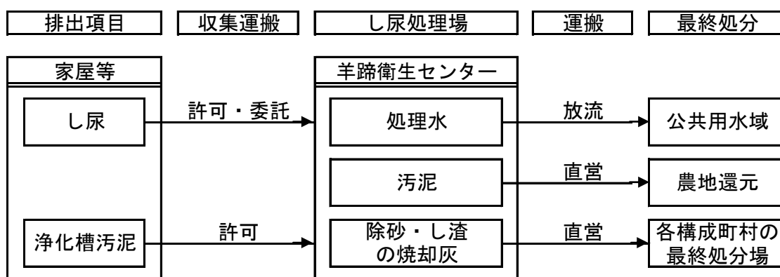
図2 し尿及び浄化槽汚泥の処理フロー
