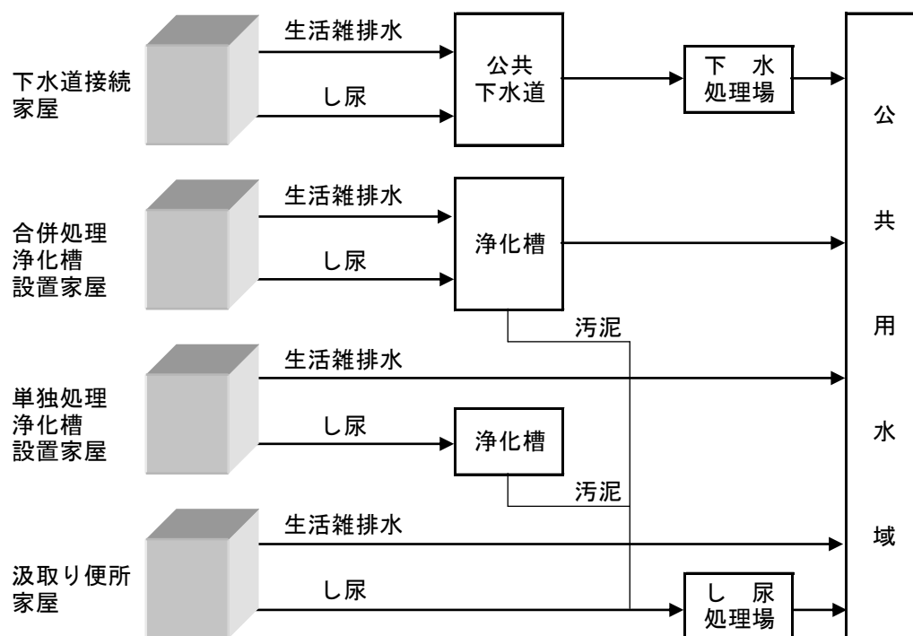
図1 生活排水の処理フロー
